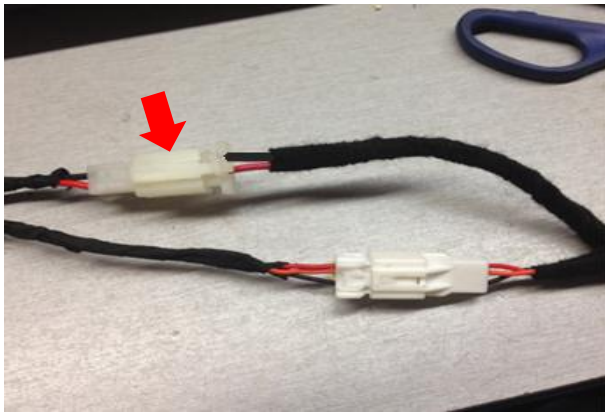
左右电机接线方法：两边接法一致，正接红色接红色，黑色接黑色（箭头）
